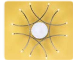
PLAFONIERA GIRANDOLA Ø cm. 52, in metallo cromato 12x10W G4 incluse
