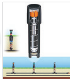
MICROIRRIGATORE COLIBRI' 90° microirrigatore a scomparsa a basso consumo d'acqua. Funzionamento ottimale anche a basse pressioni. Gittata regolabile fino a mt. 4,7. Alzo cm 5. Cod. 35840
