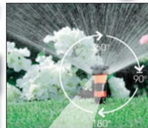
MICROIRRIGATORE COLIBRI' microirrigatore a scomparsa a basso consumo d'acqua. Funzionamento ottimale anche a basse pressioni. Gittata regolabile fino a mt. 4,7. Alzo cm 5. Disponibili per aree 180° e 360° Cod. 35838-9
