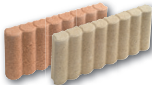
BORDURA crema e rosa, cm. 50x20x6,5 Cod. 363389-90
