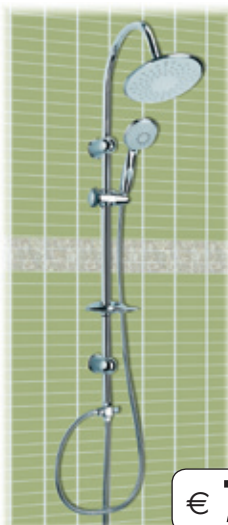
COLONNA DOCCIA in ottone cromato con doccetta anticalcare a 4 getti + pausa, soffione da cm. 20, flessibile in acciaio inox doppia graffatura. Fissaggio a muro regolabile.
