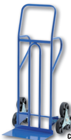
CARRELLO DA TRASPORTO in acciaio a tre ruote con pala cm. 50x30. Portata kg. 250. Cod. 357006
