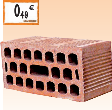
MATTONE U.N.I. DOPPIO Da intonaco, cm 12x12x25 08268
